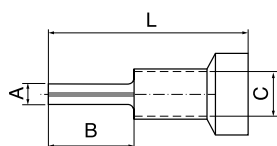
Puntale rotondo
