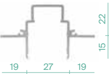
DISEGNI TECNICI TECHNICAL DRAWINGS
