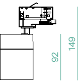
Ø 68
